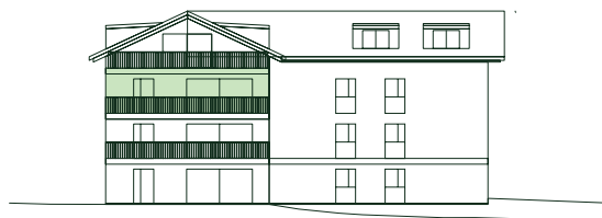
FACADE SUD-EST
