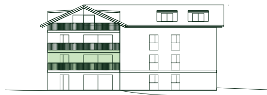
FACADE SUD-EST
