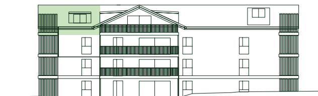
FACADE SUD-OUEST
